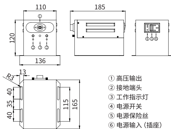
AP-AY1604 结构尺寸图
