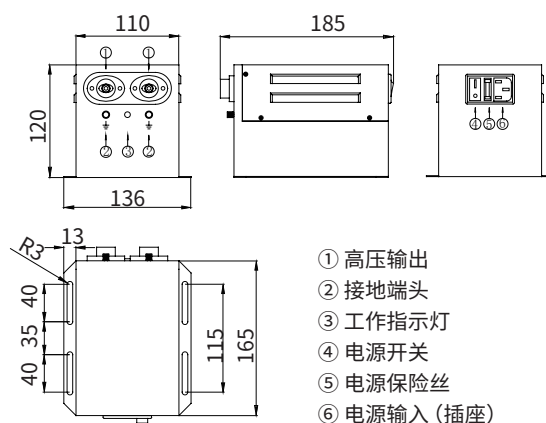
AP-AY2604 结构尺寸图
